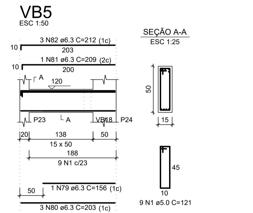
Armação Viga Escala 1:50
